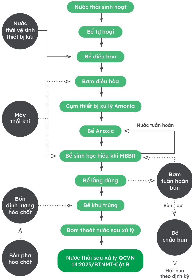
Sơ đồ xử lý nước thải tại tòa nhà văn phòng
